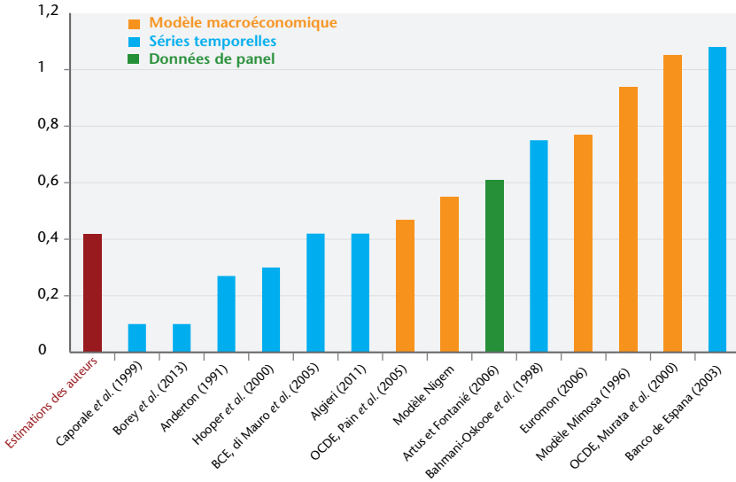
Graphique 4. Élasticité-prix des exportations pour l'Allemagne : une revue de la littérature
